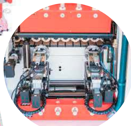
2 Motoriges Eckenkopieraggregat
