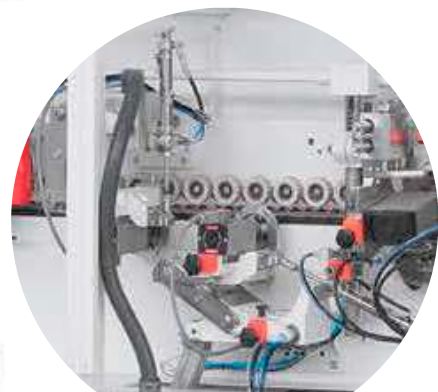
2 Motoriges Eckenkopieraggregat
