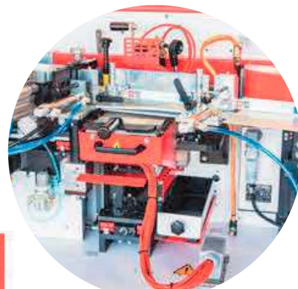
Schnellwechselleimbecken
